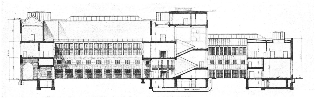
Basel, Kunstmuseum oben Längsschnitt, unten Querschnitt durch die beiden Binnenhöfe
