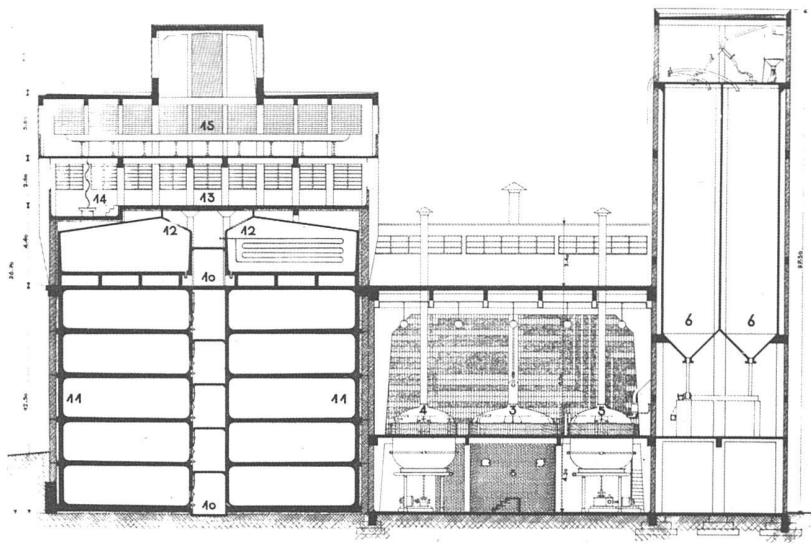
Längsschnitt 1:400
