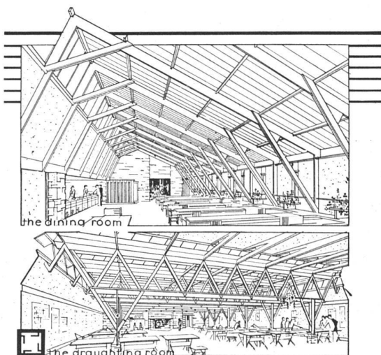
Zwei Seiten aus dem Projekt von F. L. Wright
