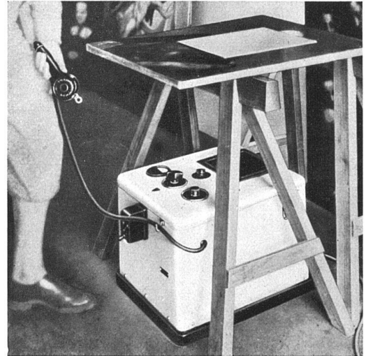
Röntgenuntersuchung eines Gemäldes Der Apparat ist mit einem automatischen Zeitschalter in der Hand des Untersuchenden verbunden. Der Film wird, ohne aus dem Umschlag genommen zu sein, auf den zu durchleuchtenden Teil des Bildes gelegt
