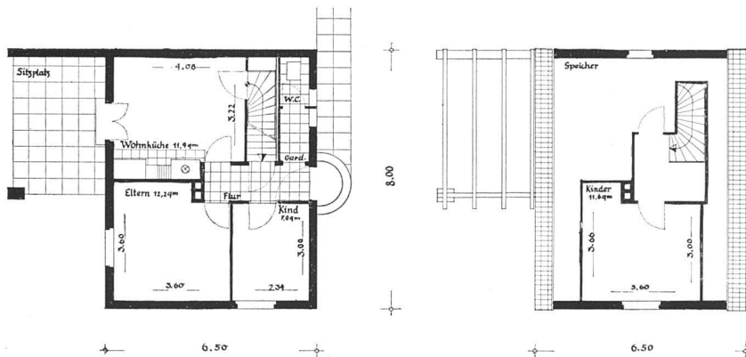
Grundrisse 1:200
