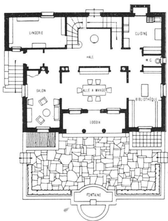
Plan rez-de-chaussée 1:300 Voir les plans du sous-sol et du 1er étage à la page suivante
