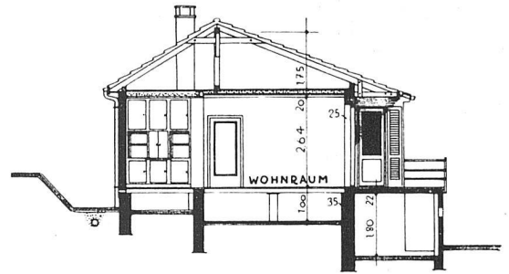
Schnitt 1:200
