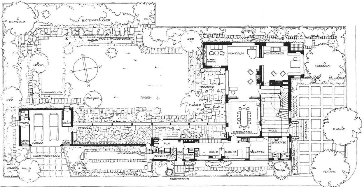
Erdgeschossgrundriss 1:400
