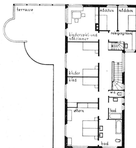
Obergeschoss 1 : 300
