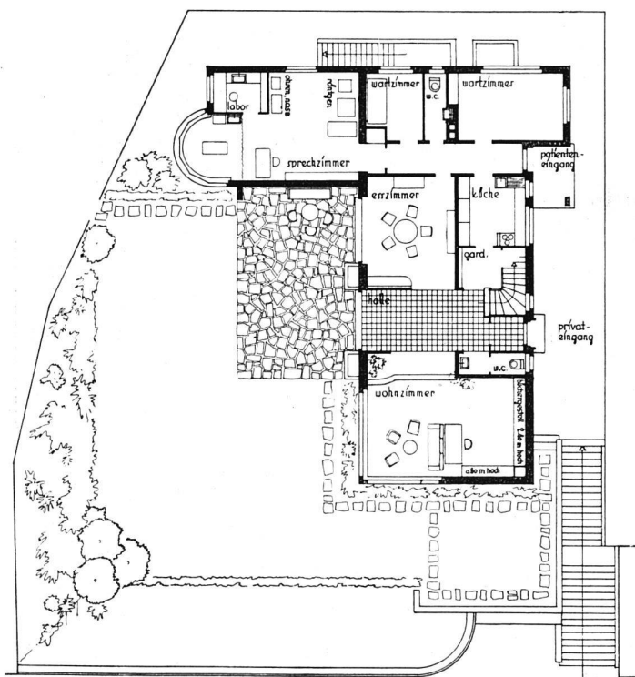
Situationsplan und Erdgeschossgrundriss 1 : 300
