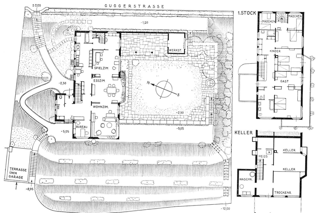
Haus Diem Zollikon (Zürich) Laubi & Bosshard, Architekten, Zürich
