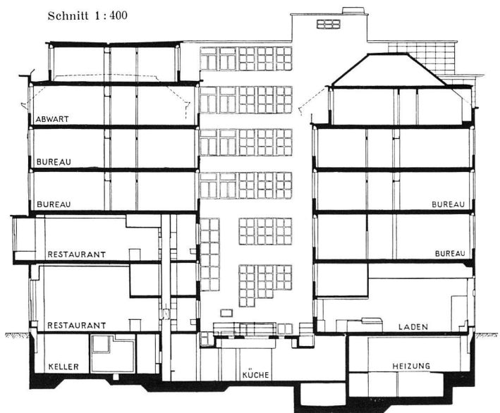
Schnitt 1:400
