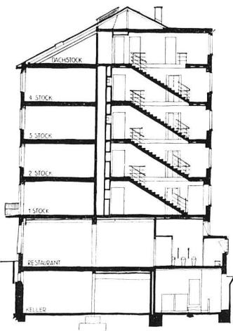
Schnitt 1:400
