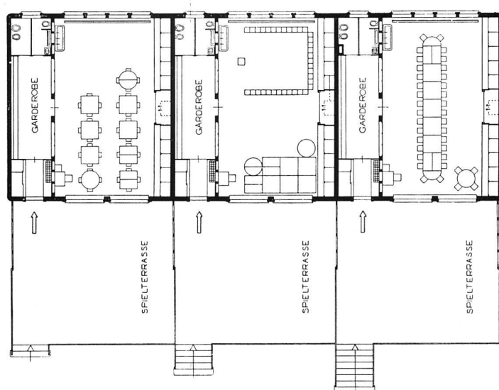
Grundrisse Keller und Erdgeschoss 1:300
