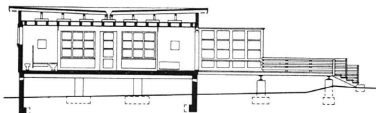
Schnitt 1:300
