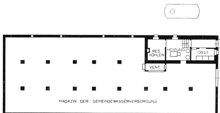
Grundrisse Keller und Erdgeschoss 1:300
