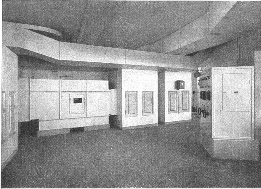
Luftkonditionierungsanlage für den neuen Rotationsmaschinenaal der Buchdruckerei Berichthaus, Zürich, verbunden mit kompletter Lüftung der Garage, Wagenwäscherei und des Speditonsraumes
