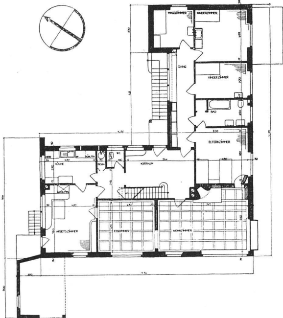
Erdgeschossgrundriss 1:300
