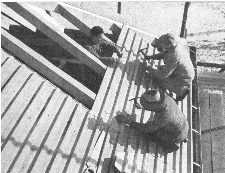
Ein Eternitrippen-Unterdach ist schnell verlegt
