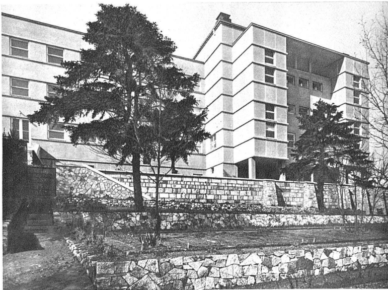
Botanisch-zoologisches Institut der Universität Istanbul, erbaut 1936
