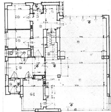
Grundriss Haus Ragip Bey 1:300
