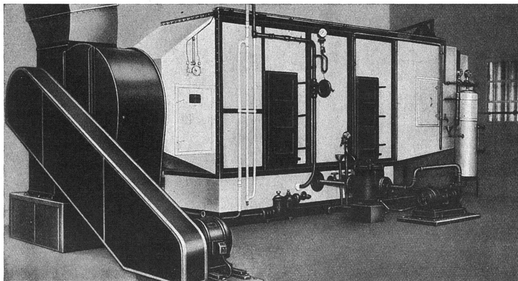
Ansicht einer Klima-Anlage (Ventilator, Luftwascher, automatische Regelapparate etc.), wie wir sie im Corso-Theater, Zürich, Kinotheater Urban und Roxy, Zürich, Bel Air Metropole, Lausanne, etc. aufgestellt haben
