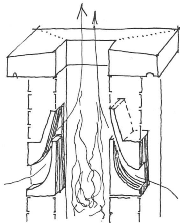
Der « Simplex-Einsatz » fördert den Zug im Kamin ohne Spezial-Hut. Ausführung durch Eugen Schädel, Güterstraße 105, Basel. Preis für das einzelne Stück Fr. 3.20.
