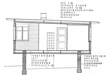
Schnitt 1:200
