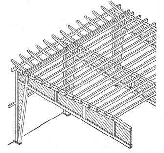
Abb. 8 Axonometrie der Holzkonstruktion mit durchlaufenden Sparren über den Rahmenbindern. Vordach mit Gegengefälle und zurückverschobener Rinne
