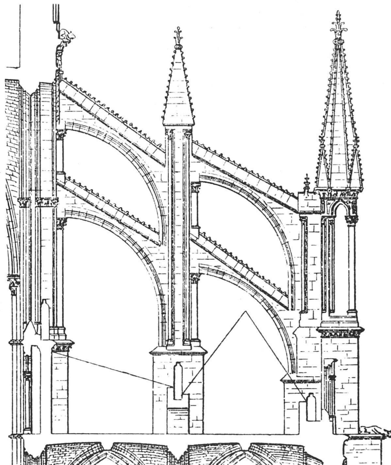
Kathedrale von Reims. Ausgeführtes Strebensystem des Chors (geweiht 1241) Nach King, The study book of mediaeval architecture
