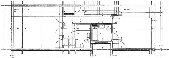
Wohnungsetage mit Kleinküche ca. 1:100
