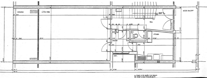
Wohnungsetage mit Kleinküche ca. 1:100
