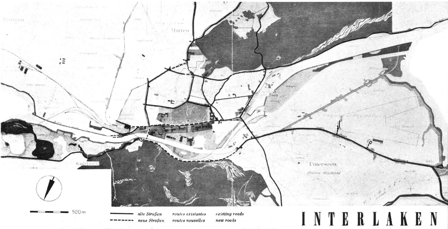
Verkehrsplan 1:30 000
