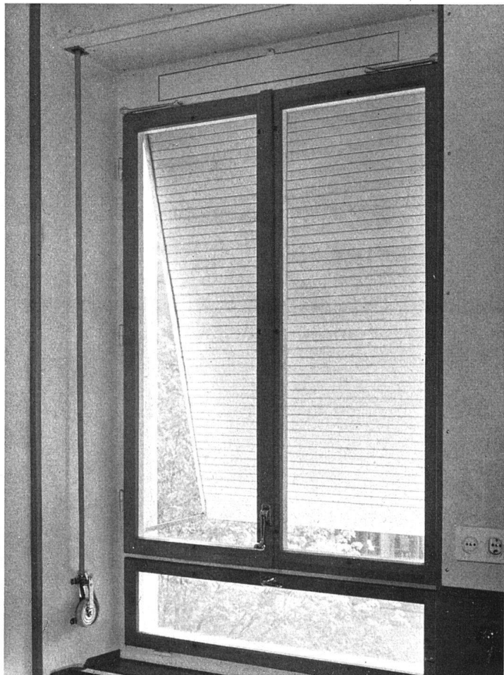
Abb. 31 Fenster von innen. Unten Querflügel, oben Lüftungsklappe. Der hellgestrichene Rolladen reflektiert das auf die weiße Fensterbrüstung auffallende Sonnenlicht. Espagnolette-Verschuß (Modell AKZ/Metallbau Koller, Basel)
