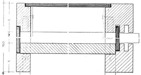
Detail 1:6 Vertikalschnitt
