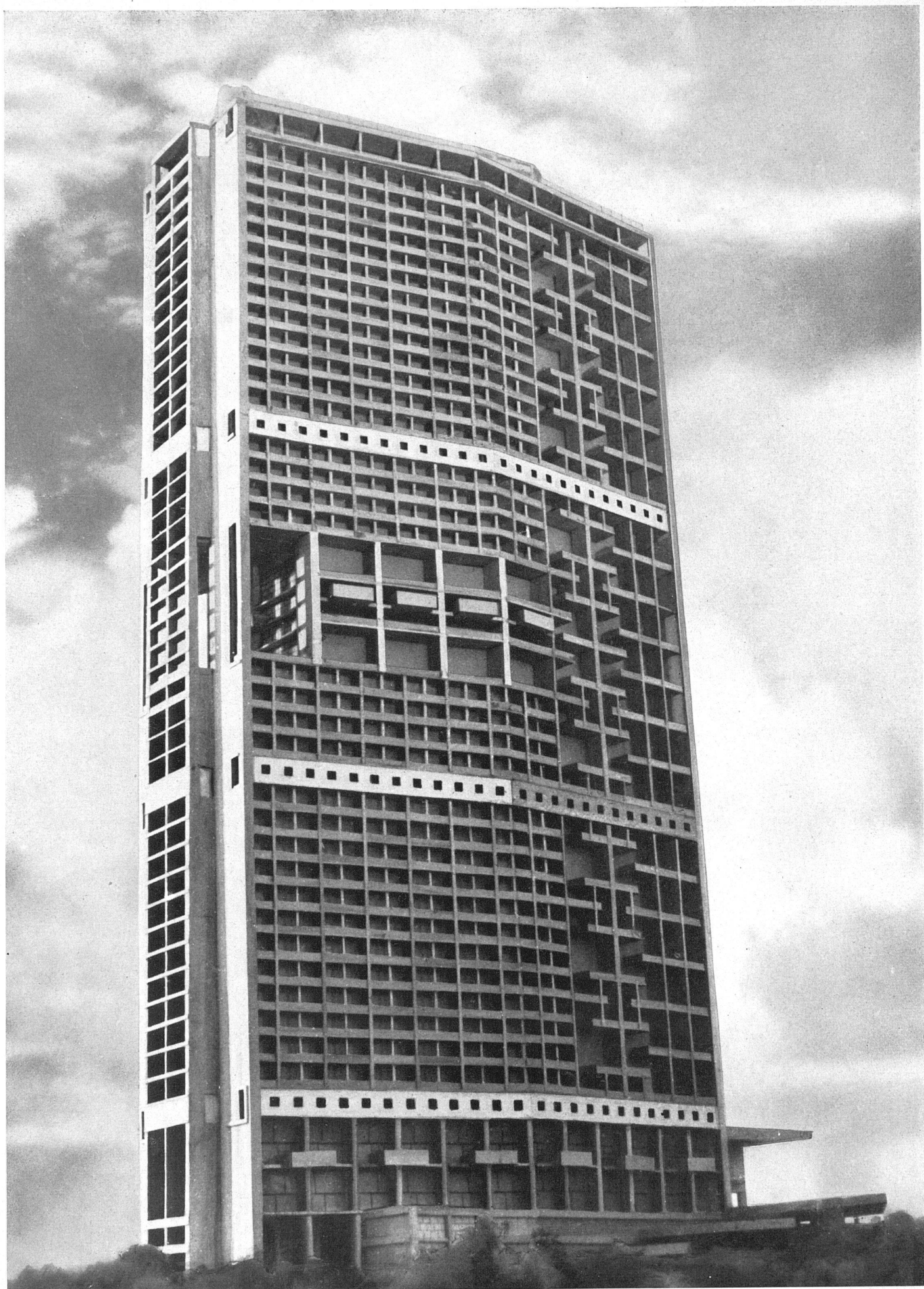
Modellansicht. Systematischer Sonnenschutz und bewußte Rhythmisierung der Fassaden / Maquette: la section d'or a fourni l'harmonie et la cadence de l'enveloppe munie de brise-soleil / Harmony and rhythm of the shell with its «brises-soleil» resulted from the application throughout of the golden-rule
