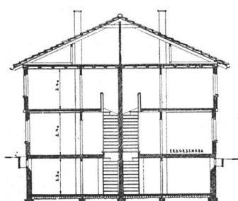
Schnitt Einfamilienhaus Coupe / Section
