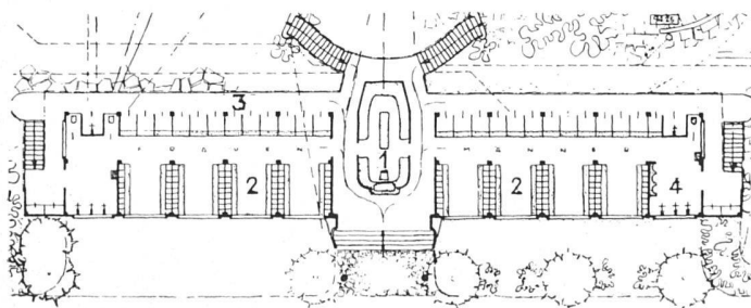
Garderobengebäude 1:300, Erdgeschoß / Bâtiment des vestiaires, rez-de-chaussée / Cloakroom building, ground floor
