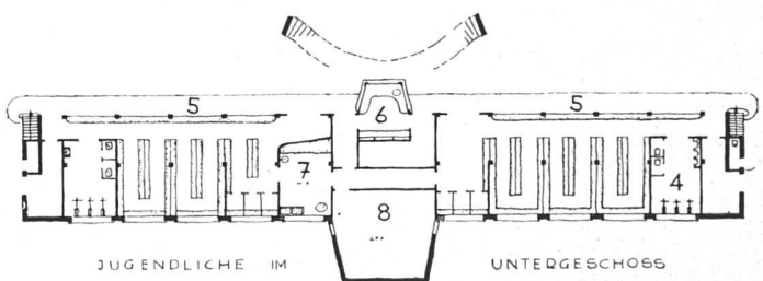
Untergeschoß für Jugendliche 1:300 / Sous-sol, vestiaires scolaires / Basement floor for children
