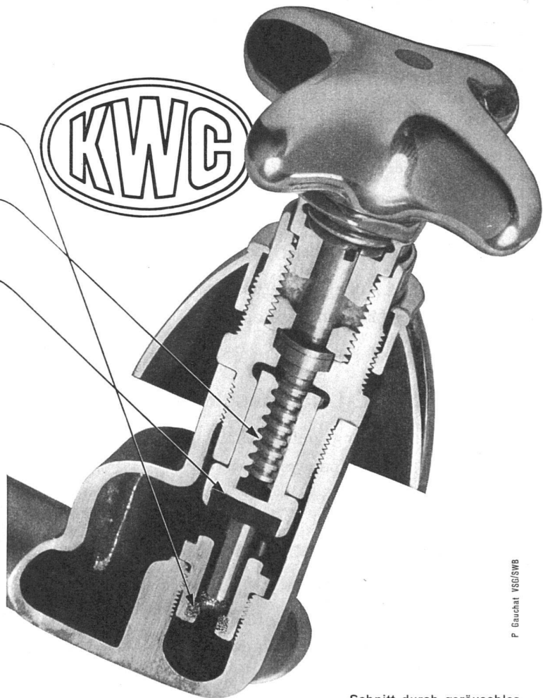
Schnitt durch geräuschlos funktionierenden Hahn
