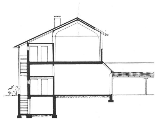
Querschnitt 1:300 / Coupe transversale / Cross section
