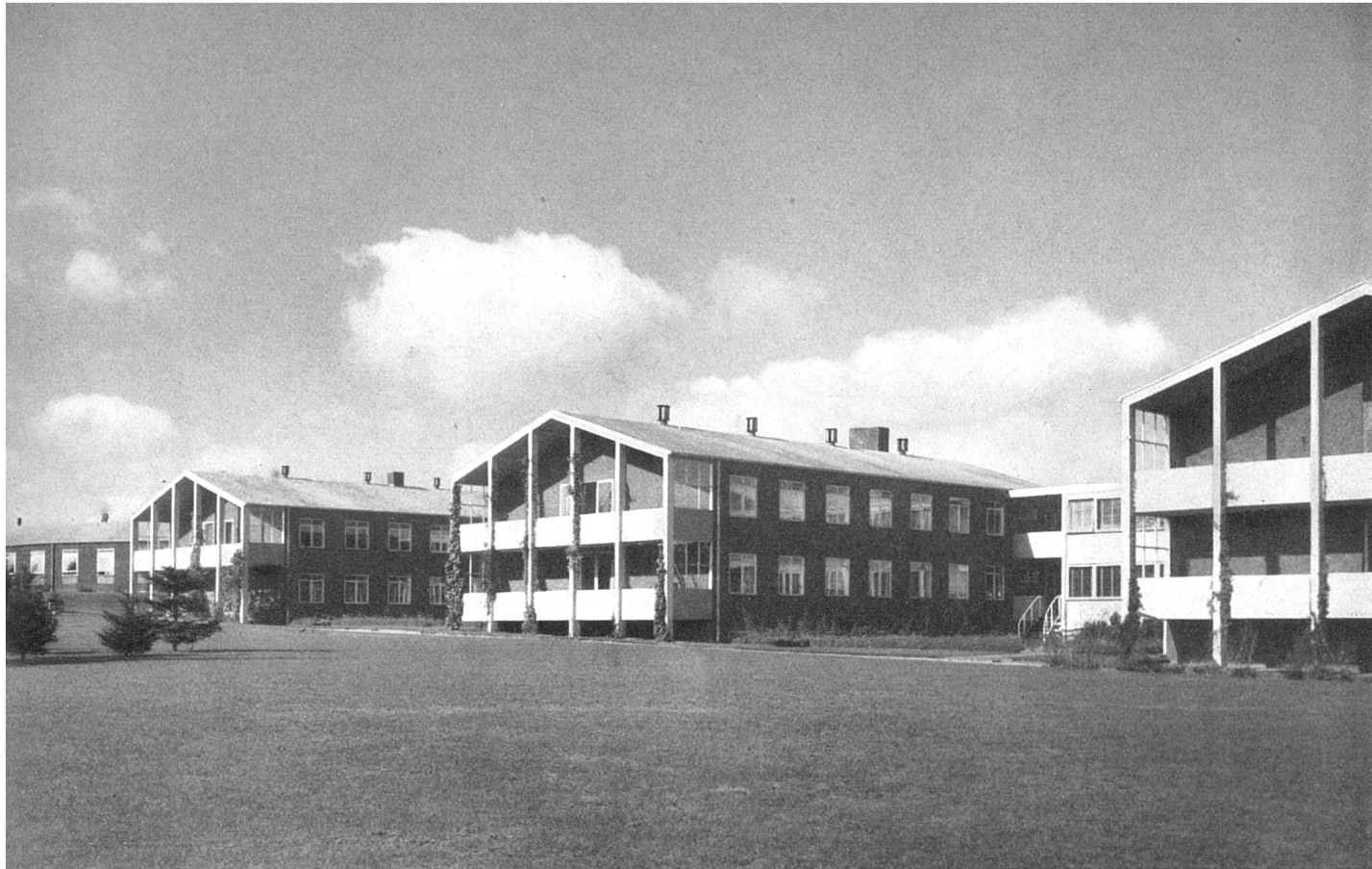
Ansicht von Süden, Wohntrakte mit Giebelterrassen / Vue d'ensemble (sud); maisons d'habitation avec balcons / General view from the south, dormitories with balconies Photo: Maarbjerger Atelier, Kopenhagen
