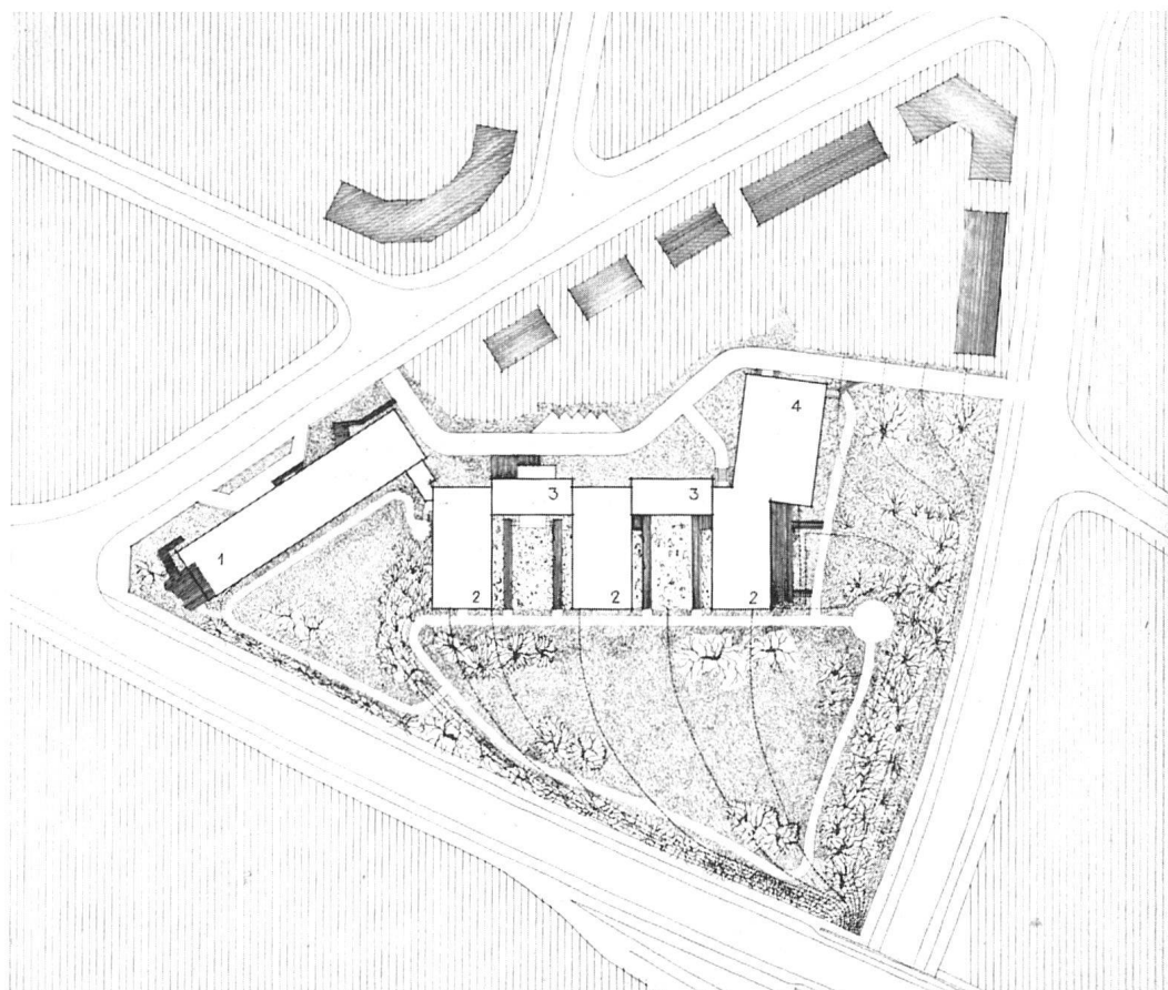
Situation I: 2000 / Plan de situation / Site plan
