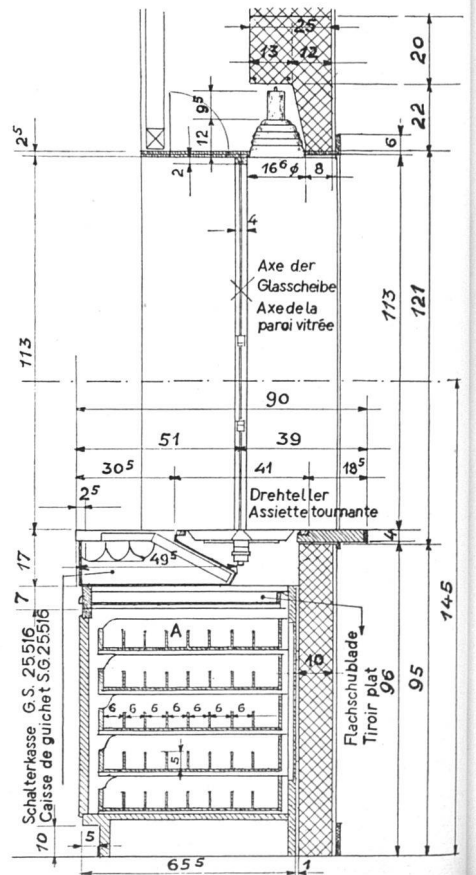
Schnitt durch Billettschalter / Coupe du guichet / Section through ticket window
