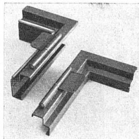
norm Türzargen
