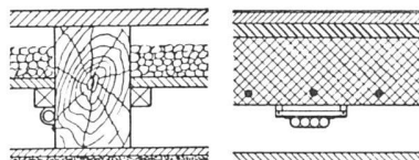
Leitungsverlegung in Holzbalkendecken
