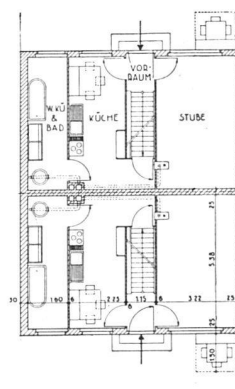
Abb. 10. Erdgeschoß 1:300 | Rez-de-chausée | Ground floor plan
