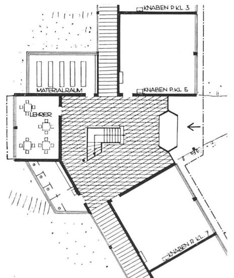
Erdgeschoß mit Eingang 1:400 | Rez-de-chaussée et entrée | Ground-floor plan with entrance
