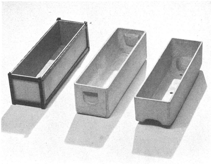
Entwicklung des Blumenkistchens. Links: Eisengestell mit Eternitplatten ohne Griff; Mitte: Ganzeternitkästchen mit Griff; rechts: verbessertes neues Modell mit gutem Griff | Trois phases successives du casier fleurs; à droite, le dernier modèle | Three stages of the development of the flower box, at right, the new type
