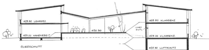
Klassenzimmer 1:400 | Salles de classe | Classrooms
