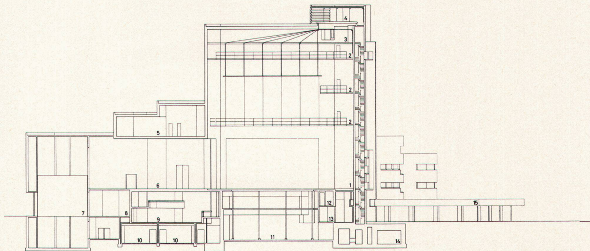
10 Schnitt quer zur Bühnenachse Coupe sur l'axe transversale de la scène Section across the transversal stage axis
