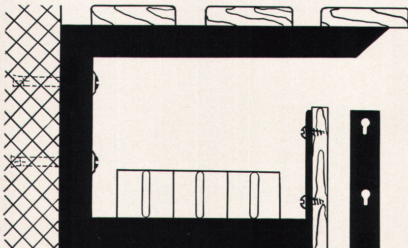
Sitzbank-Konsole mit Konvektorenträger. Frontverschalung auf Bajonettverschluß. Wand- oder Bodenverankerung. Richtpreis Fr. 12.— bis 15.— einbrenngründiert
