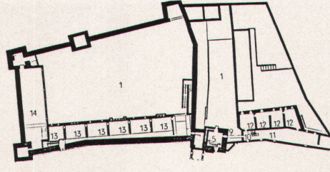
2 Plans rez-de-chaussée, premier et second étage du Musée municipal de Castelveccchio, Vêrone
