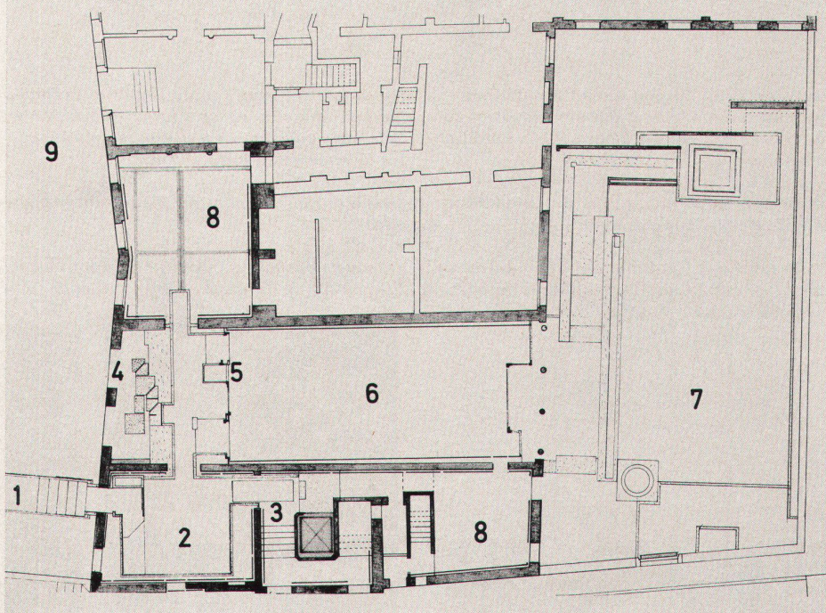
1 Grundrisse Erdgeschoß der Stiftung Querini Stampalia, Venedig; oben: vor dem Umbau; unten: nach dem Umbau
