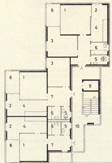
GRUNDRISS INVALIDENWOHNUNGEN 6
