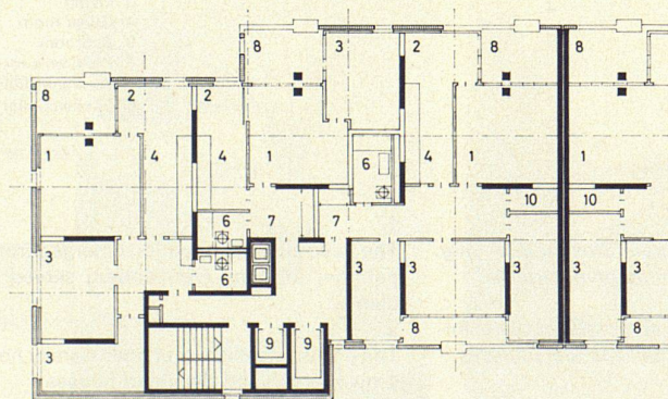
GRUNDRISS WOHNHOCHHAUS 5
