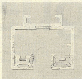
solide Leichtmetall-Stromschiene
