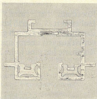
Stromschiene mit Flanken für herabgehängte Decken
