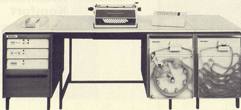
Addo-Forster 2500 – ein Korrespondenz- und Organisations-Automat für integrierte Arbeitsabläufe ab Lochstreifen, Lochstreifen-Karten und Lochkarten. Eine logische Konzeption in der Datentechnik.
