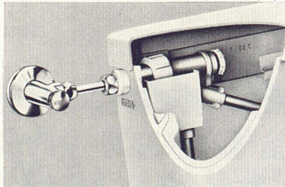
Die bewährte GEBERIT-Vollisolation gegen Schwitzwasserbildung.
