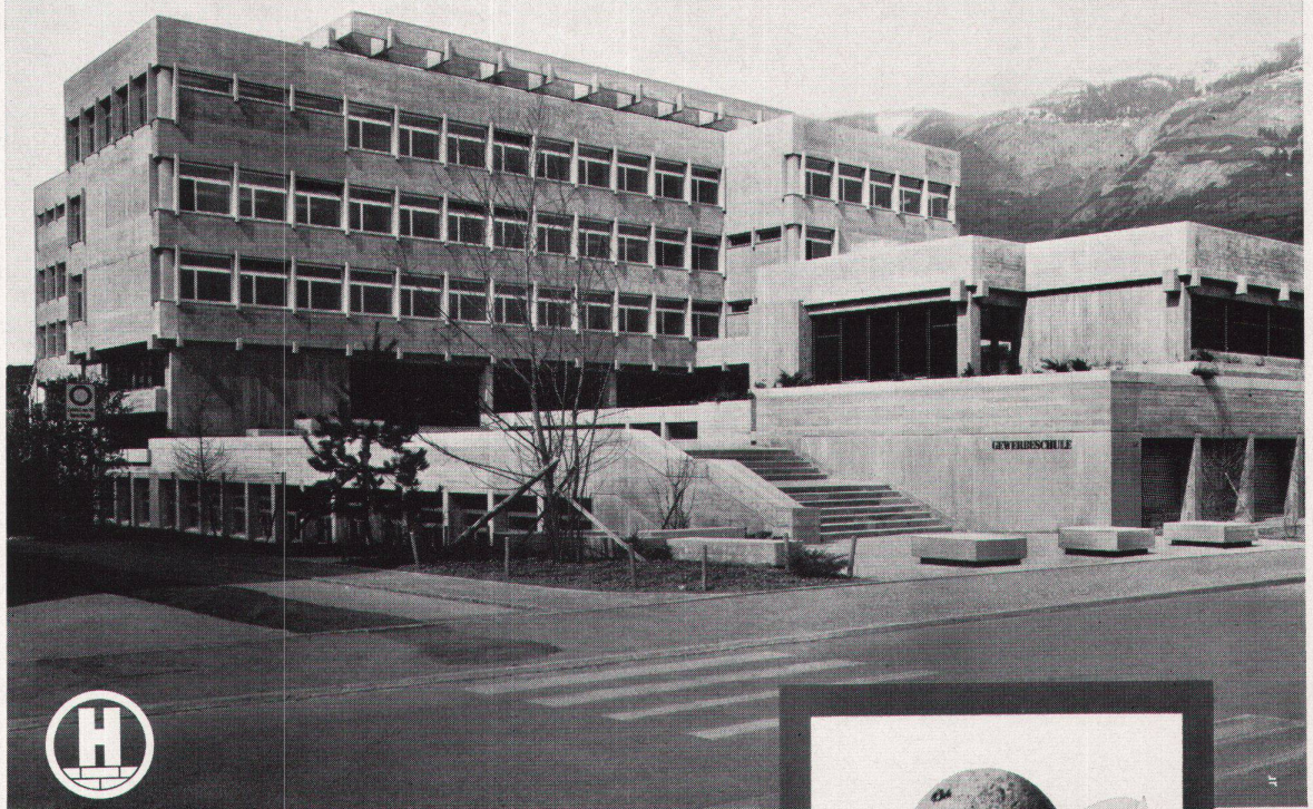
Gewerbeschulhaus Chur; seine Fassaden und Dachaufbauten sind —teils an Ort geschüttet, teils vorfabriziert— in Leca - und Normalbeton ausgeführt. Planung: A. Liesch, dipl. Architekt BSA/SIA Statik: Jenatsch + Hegland, Ingenieure, Chur
