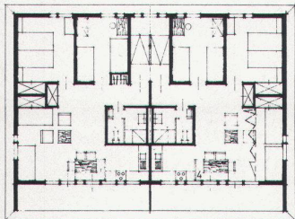
Grundriss 1. Obergeschoss Plan du premier étage
