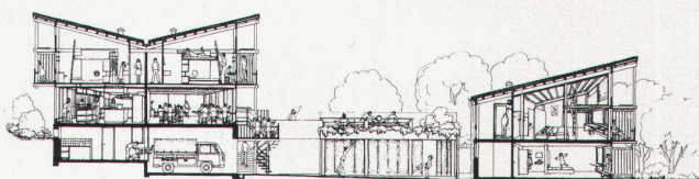
Schnitt BB Coupe BB
