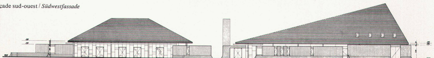
Façade sud-ouest / Südwestfassade
