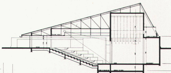
Coupe / Schnitt AA
