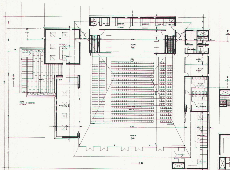
Plan / Grundriss
