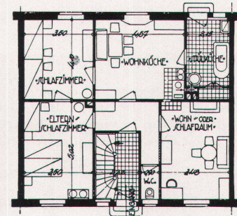
8 Grundriss einer 4-Zimmer-Wohnung
